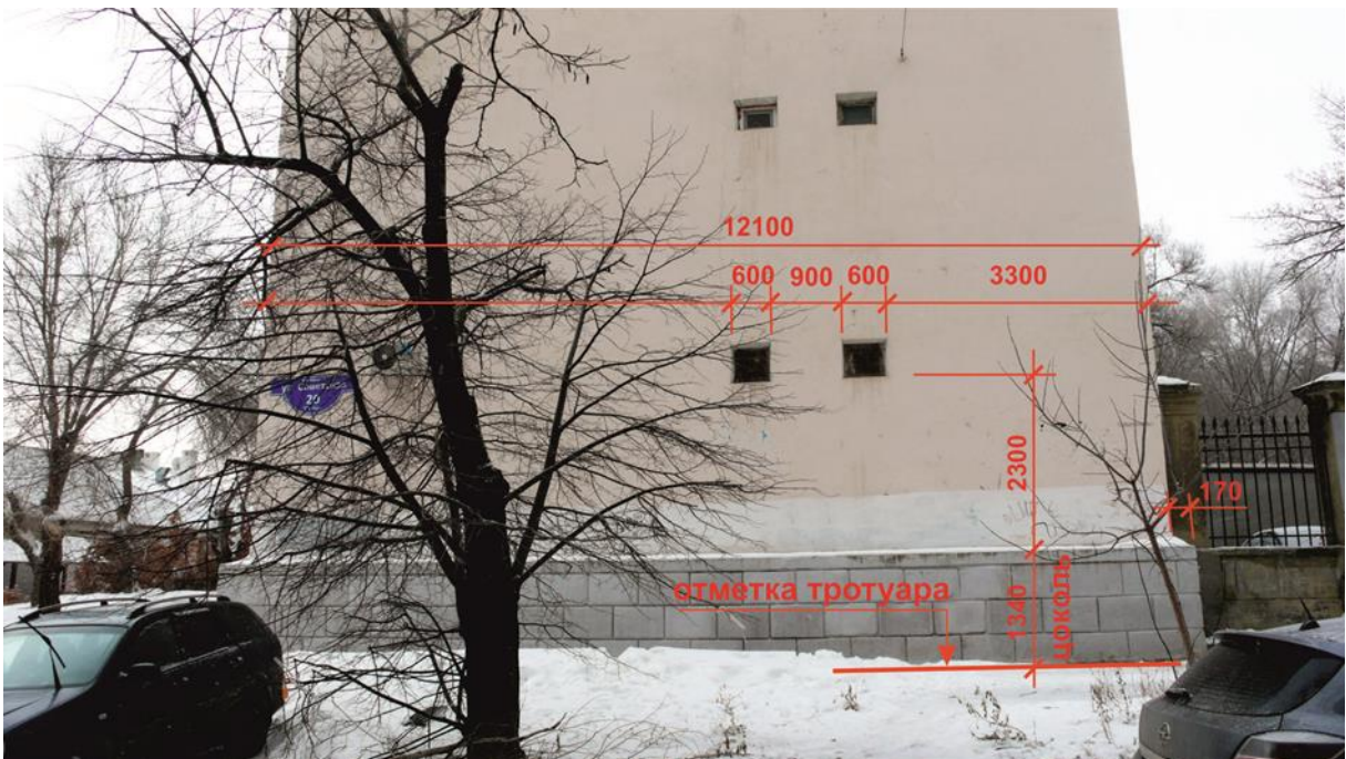
Рис. 15. Корпус «А» дома специалистов. Основные размеры участка фасада здания, где предполагается установка памятных досок
